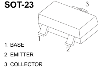
SOT-23
