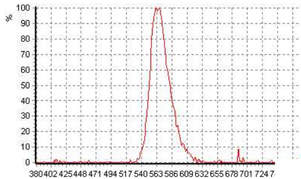
相对光谱分布曲线 (绿色) Relative Spectral Distribution Curve
