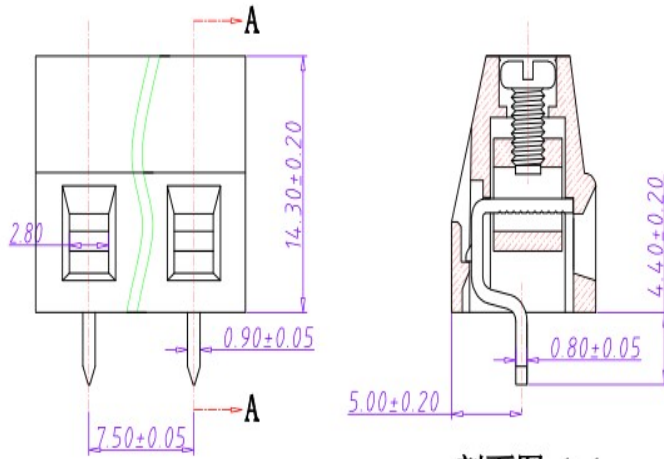
剖面图 A-A
