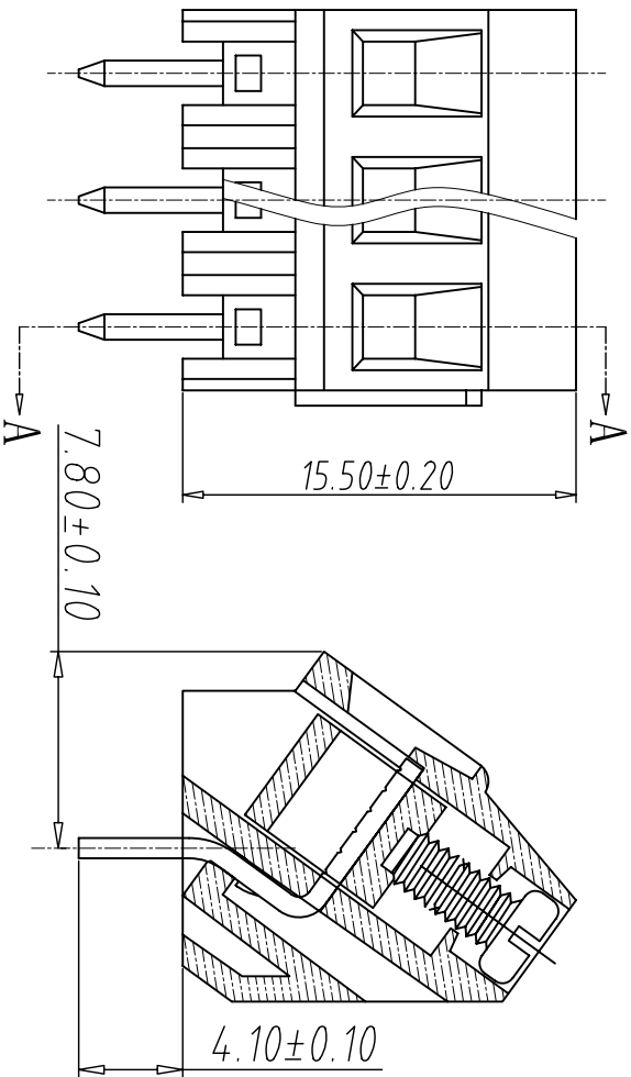
剖面图 A-A
